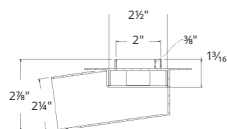
Section B-B FFTIF 65
